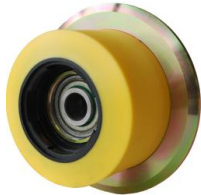
121001441 Afm.: 95 x 55 Flens: 130 (Staal) Open As M16
