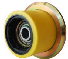
121001244 Afm.: 75 x 55 Flens: 105 (Staal) Open As M16
